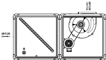
Montagem Horizontal/Descarga Vertical
