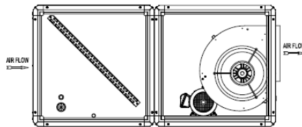
Montagem Horizontal/Descarga Horizontal
