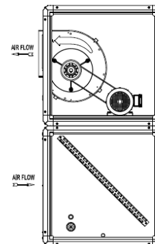
Montagem Vertical/ Descarga Horizontal Frontal
