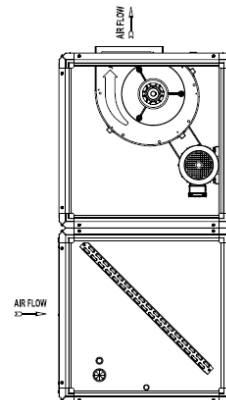
Montagem Vertical/ Descarga Vertical
