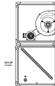
Montagem Vertical/ Descarga Horizontal Traseira
